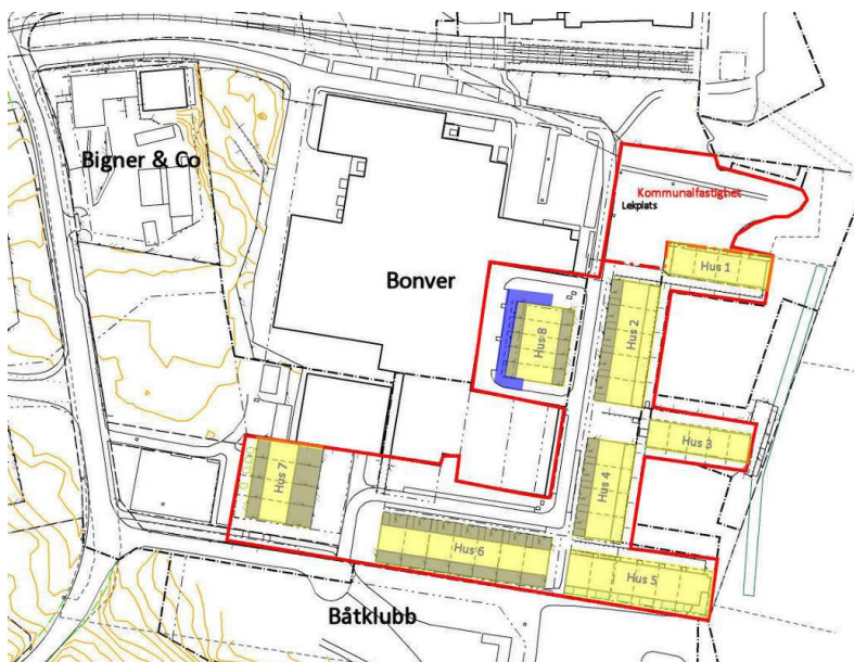
Figur 1. Område som omfattas av markundersökningen och den fördjupade riskbedömningen. Gulmarkerade områden visar separata fastigheter. Gråmarkerade partier visar uteplatser med underlagrande jord. Lekplatsen och gräsytan i norra delen av området utgör kommunal mark. Blått visar området med förhöjda halter PAH vid Hus 8.
